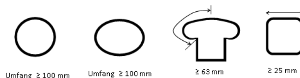
Abb. 3: Beispiele Sitzstangen
