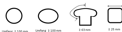
Abb. 3: Beispiele Sitzstangen
