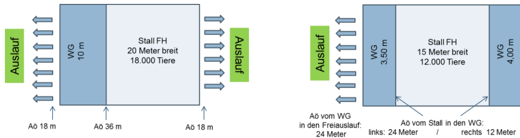
Abb. 1: Beispielskizze Auslauföffnungen / Zugänge Stall &amp; KSR
